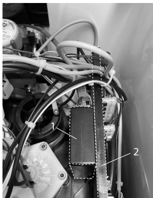
Abb. 14: Connectivity-Modul in Halterung
