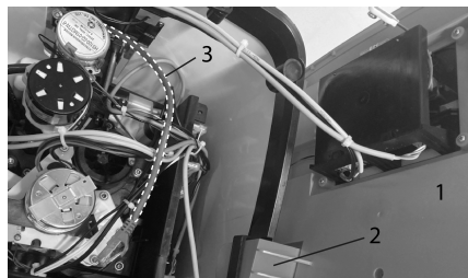
Abb. 12: LAN-Kabel durch Rückwand geführt
