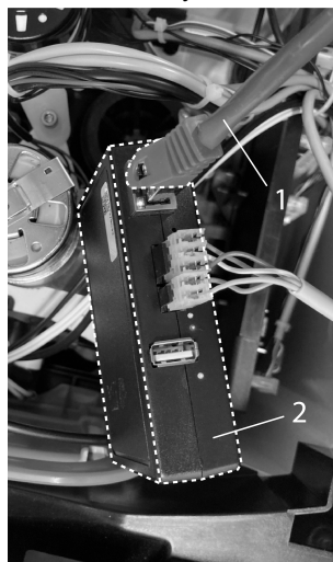
Abb. 13: LAN-Kabel am Connectivity-Modul einstecken
