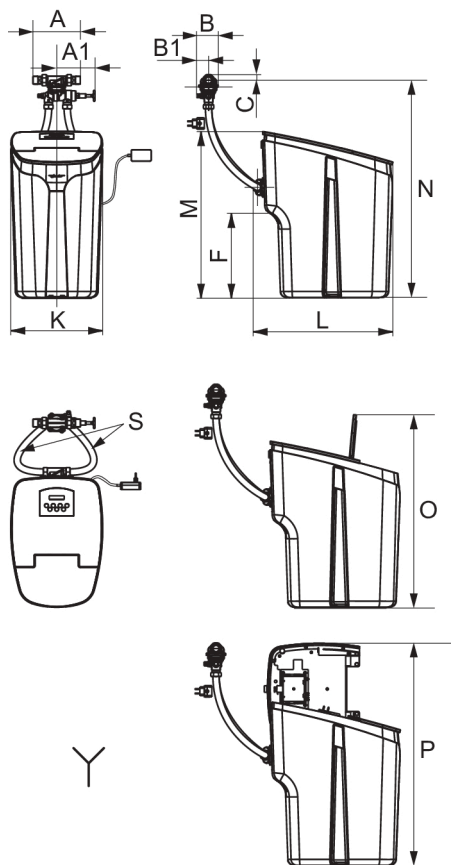
Abb. 15: Einbaumaße i-soft K
